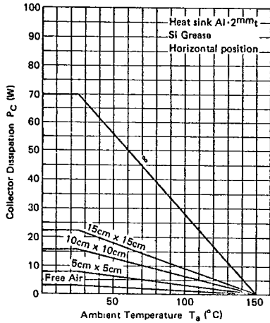
Pc - Ta
